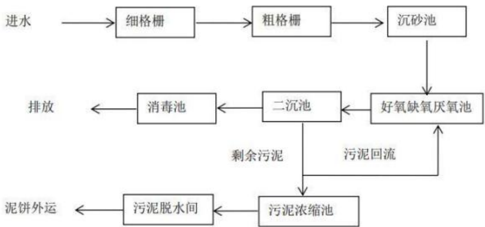
图 4-4 东海县驼峰乡污水处理厂处理工艺流程图
