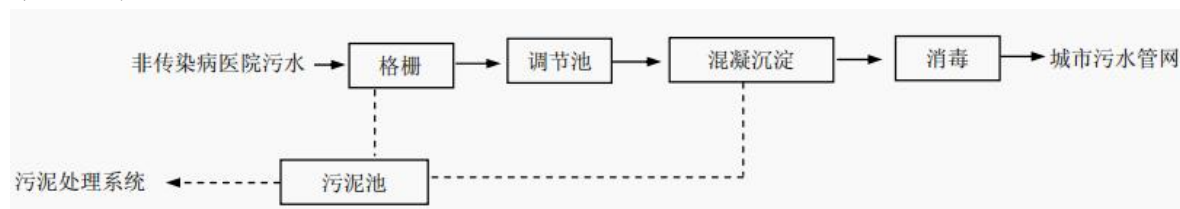
图4-3 非传染病医院污水一级强化处理工艺流程
